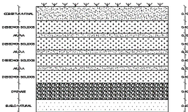
Gráfico 16 Esquema del funcionamiento de la celda emergente:
